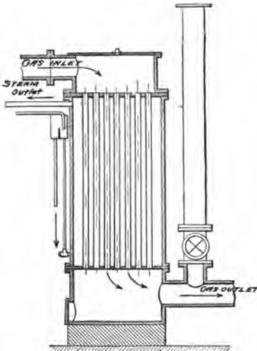
FIG. 85.—Vaporizer.
